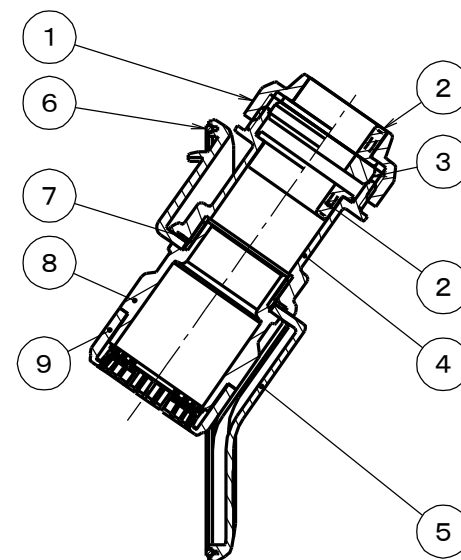
A-A断面図
